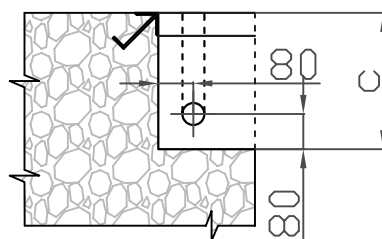
вывод кабельного канала в приямок
