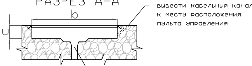
дренажное отверстие. Выполнить дренаж при установке подъемного стола вне помещения.
